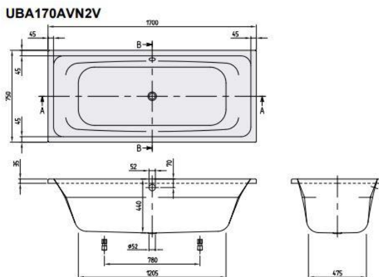
Obr. 15 - Vana rozměry
