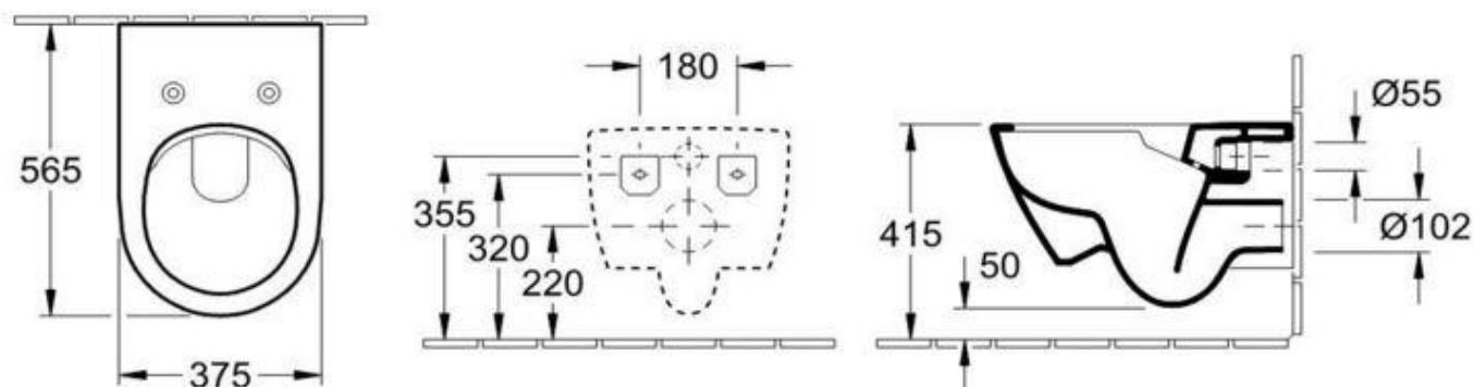
Obr. 13 – Rozměry závěsného klozetu
