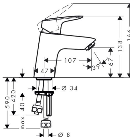
Obr. 18 - Rozměry umyvadlové baterie Logis70
