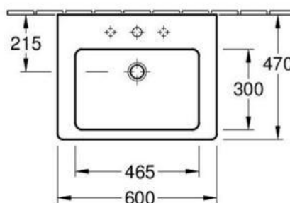
Obr. 4 – Rozměry umyvadla
