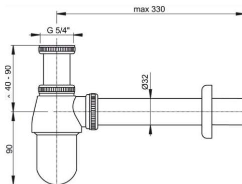
Obr. 8 – Rozměry sifonu
