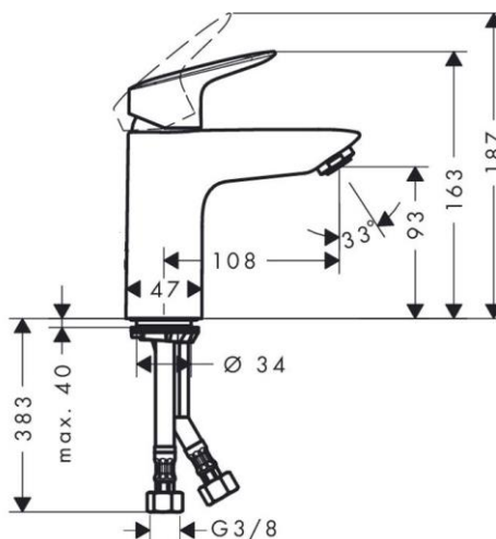
Obr. 20 - Rozměry umyvadlové baterie Logis 100
