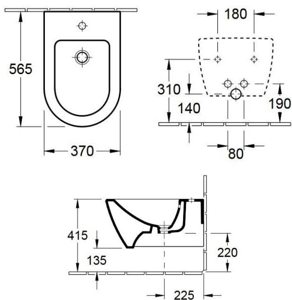
Obr. 10 – Rozměry závěsného klozetu
